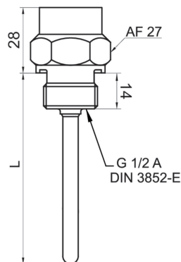
G 1/2 A DIN EN ISO 1179-2 (3852-E) (G51)
