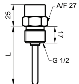
G 1/2 A ISO 228-1 (BCID: G06)
